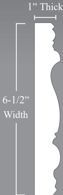
FRZ-430D-3
