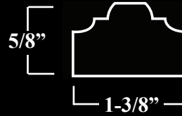
MLD-164L Profile
